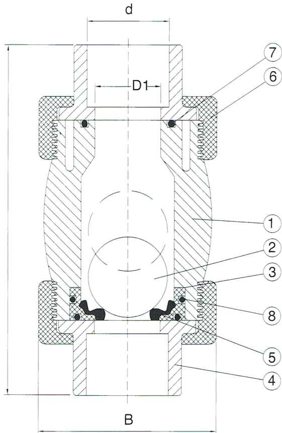
DN15~DN100
